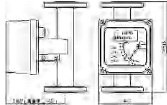
标准型 M4 指示器
