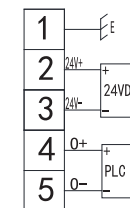
四线制供电型
